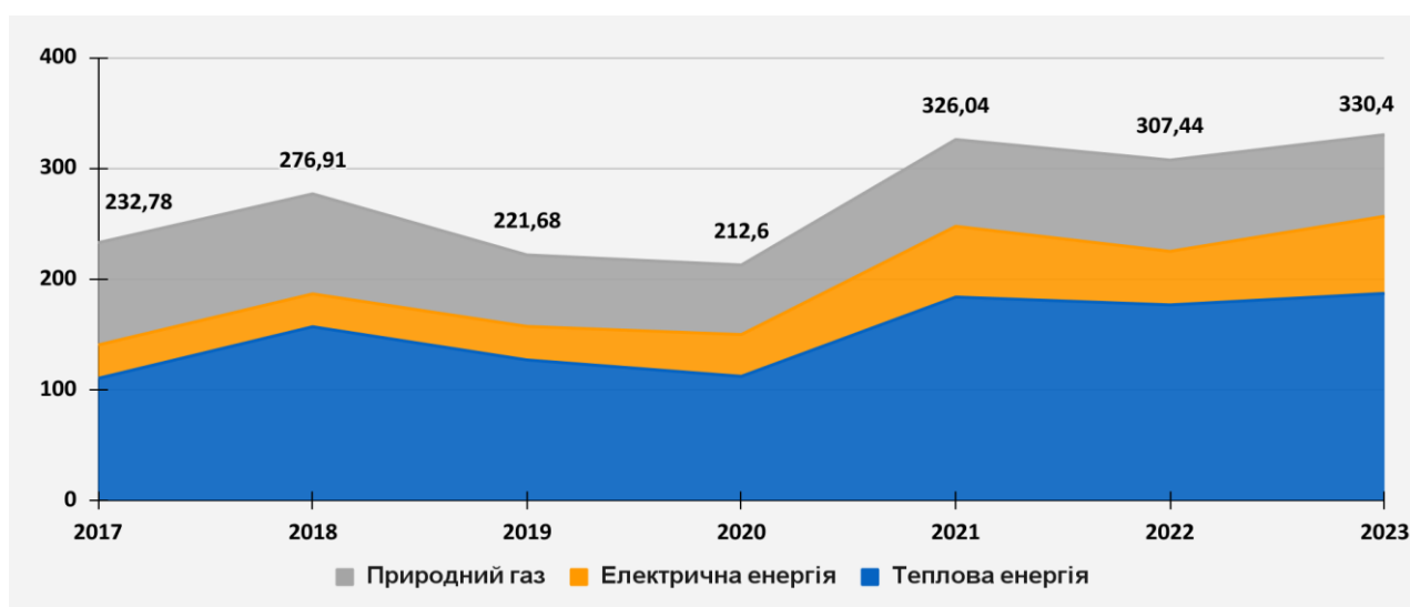
Рисунок 2.21 Вартісний баланс у секторі багатоквартирних житлових будівель, млн грн
