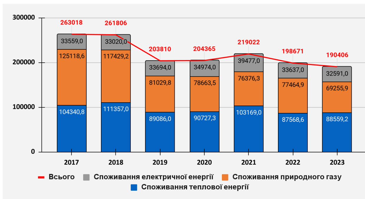
Рисунок 2.15 Споживання енергії за видами ресурсів сектором багатоквартирних житлових будівель, МВт·год
