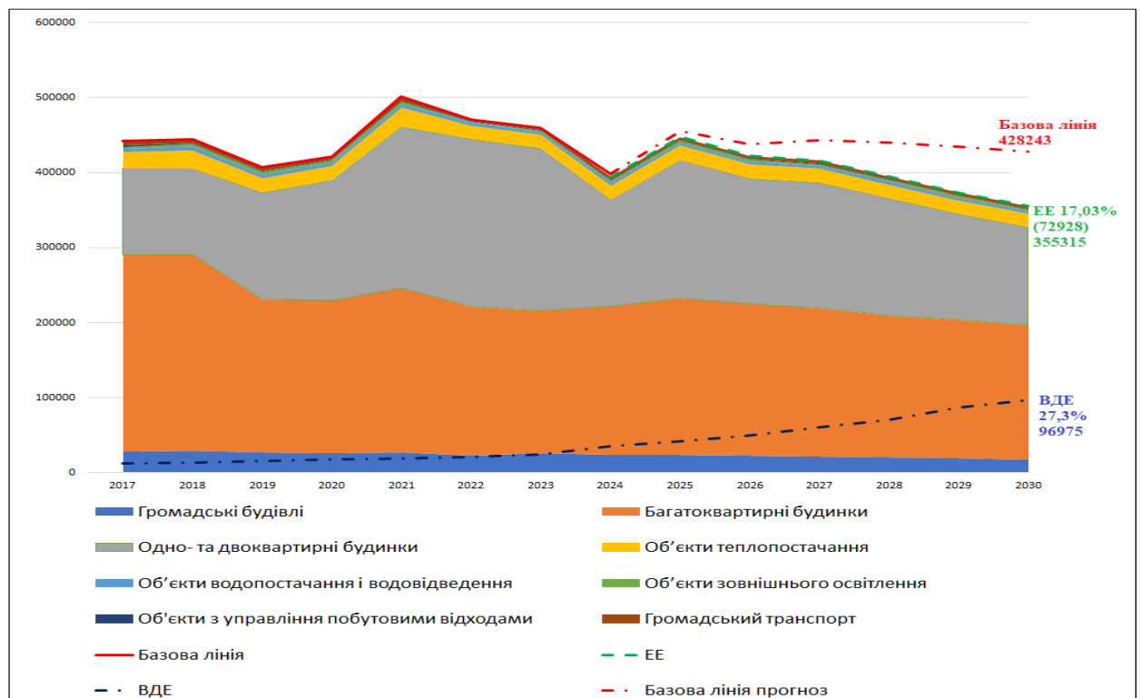
Рисунки 3.13. Базова лінія та цільові показники сталого енергетичного розвитку громади, МВт*год
