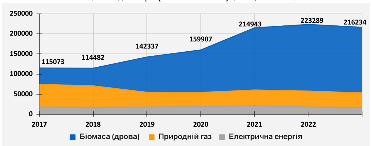
Рисунок 2.18 Енергетичний баланс у секторі одно- та двоквартирних житлових будівель, МВт·год
