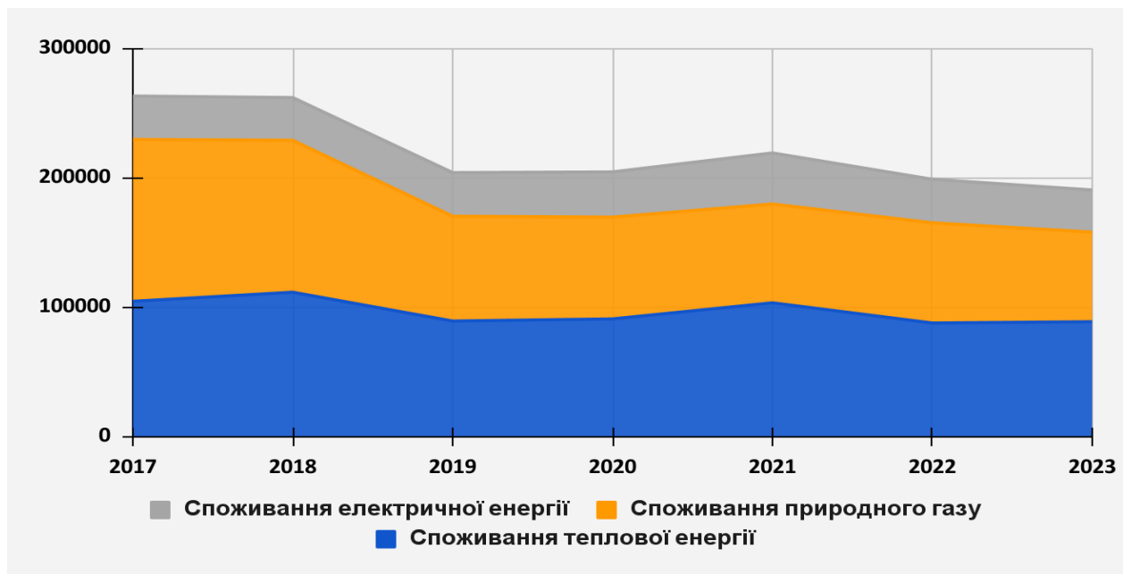
Рисунок 2.16 Енергетичний баланс у секторі багатоквартирних житлових будівель, МВт·год
