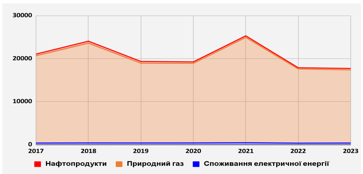
Рисунок 2.34 Загальний енергетичний баланс сектору теплопостачання, МВт·год
