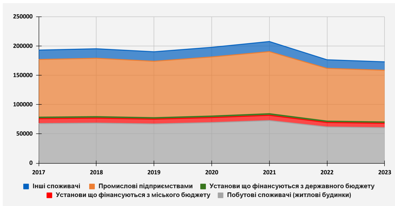
Рисунок 2.25 Споживання електричної енергії по групах споживачів, МВт*год
