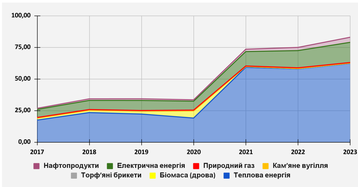
Рисунок 2.11 Загальний вартісний баланс в секторі громадські будівлі, млн грн
