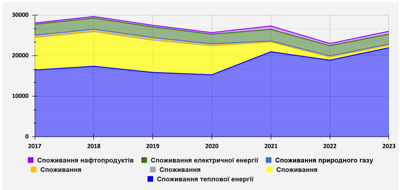
Рисунок 2.10 Загальний енергетичний баланс сектору громадські будівлі, МВт·год
