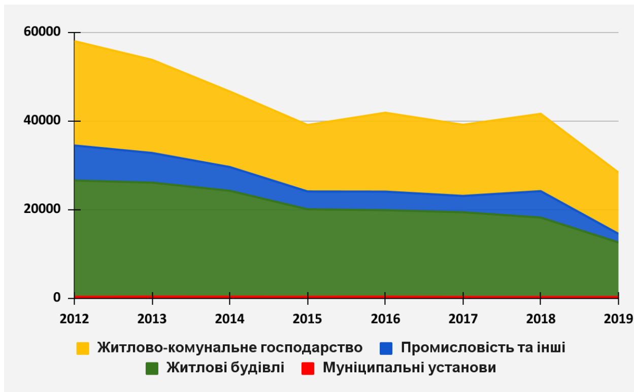
Рисунок 2.28 Споживання природного газу по групах споживачів м. Коростень за період 2012-2019 років, тис.м 3
