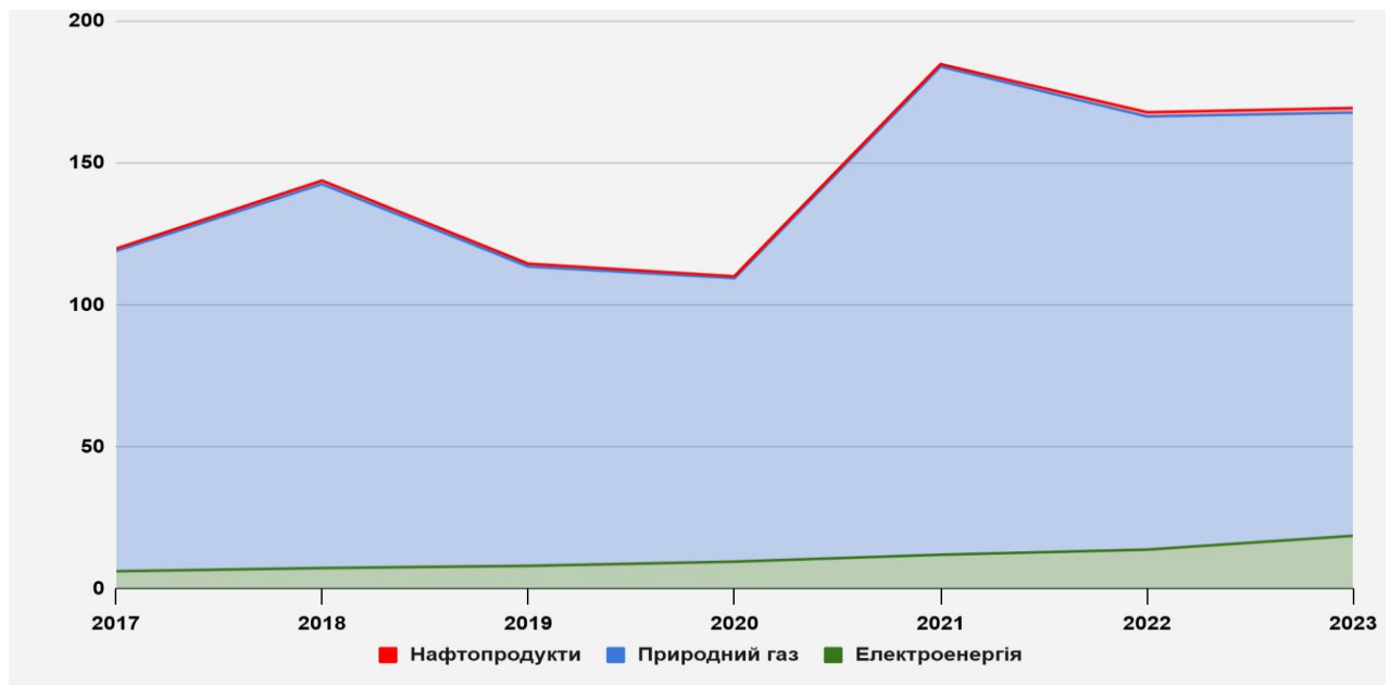
Рисунок 2.35 Загальний вартісний баланс в секторі теплопостачання, млн грн
